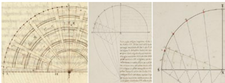
Figura 3. Ricostruzione spaziale dell'impostazione delle dimensioni dei lacunari della cupola.
