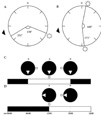
Fig. 1 - Rappresentazioni schematiche degli esperimenti di orientamento solare in Talitrus saltator A, B, rappresentazione dei saggi di deflessione dell'azimut solare, A, orientamento degli individui sagggiati in condizioni naturali, B, orientamento degli animali sagggiati in corrispondenza di azimut solare deflesso di 100^\circ in senso antiorario. N: nord, triangolo nero: direzione attesa degli individui nella spiaggia di origine; triangolo bianco: direzione attesa in base alla deflessione del sole; freccia nera: direzione media assunta dagli individui; il simbolo del sole rappresenta l'azimut solare all'ora degli esperimenti. C, D, rappresentazione dei saggi effettuati con individui sottoposti a regimi di illuminazione differenti, C, rilasci di individui sottoposti a fotoperiodo in fase con quello naturale, D, rilasci di individui sottoposti a fotoperiodo posticipato di 6 ore rispetto a quello naturale. N: nord, triangolo bianco: direzione media attesa; le barre sottostanti le distribuzioni corrispondono alle ore di luce/buio del fotoperiodo soggettivo, il simbolo del sole rappresenta l'azimut solare all'ora degli esperimenti (da Pardi, Papi 1953, doi: 10.1007/BF00350802; Pardi, Grassi 1955, < http://dx.doi.org/10.1007/BF02161321 >, modificate)
