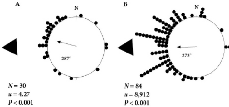
Fig. 2 - Esperimenti effettuati per saggiare l'impiego del gradiente di intensità luminosa A, rilasci in condizione di sole e cielo naturali visibili, B, rilasci sotto la cupola traslucida in Plexiglas. N: direzione del nord, pallini neri esterni alle distribuzioni: direzioni assunte da ciascun individuo, triangolo nero: direzione attesa, freccia nera: vettore medio rappresentante la direzione media assunta dagli individui, N: numero di individui, u : valore del V-test con relativo livello di probabilità ( P ) (da Ugolini, Galanti, Mercatelli 2009, < http://dx.doi.org/10.1016/j.anbehav.2008.09.035 >, modificata)
