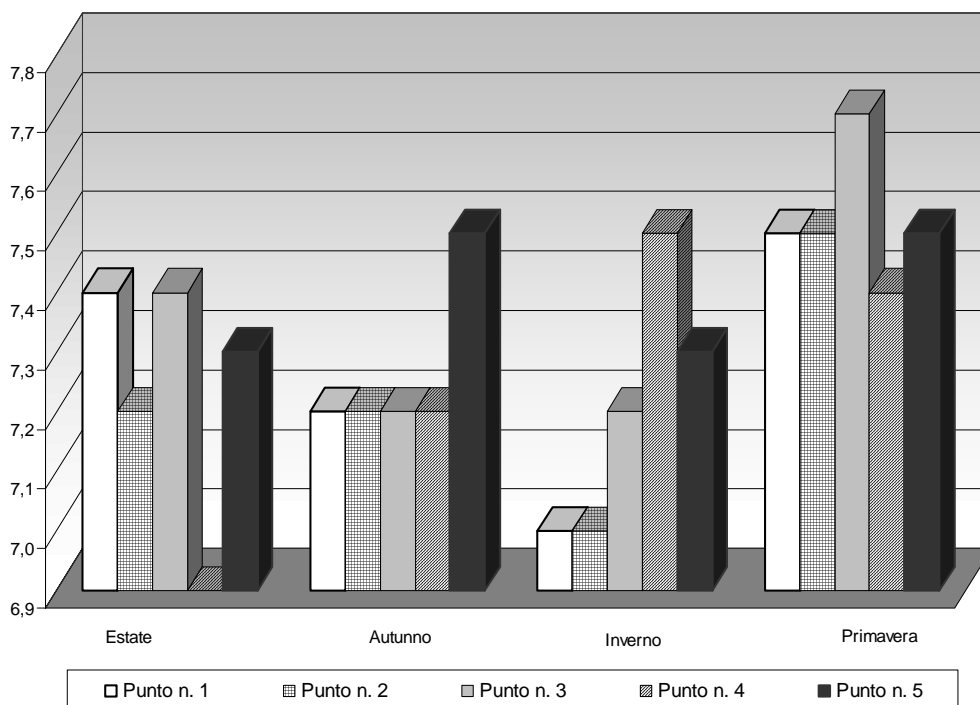
Grafico 4 - Andamento del pH.
