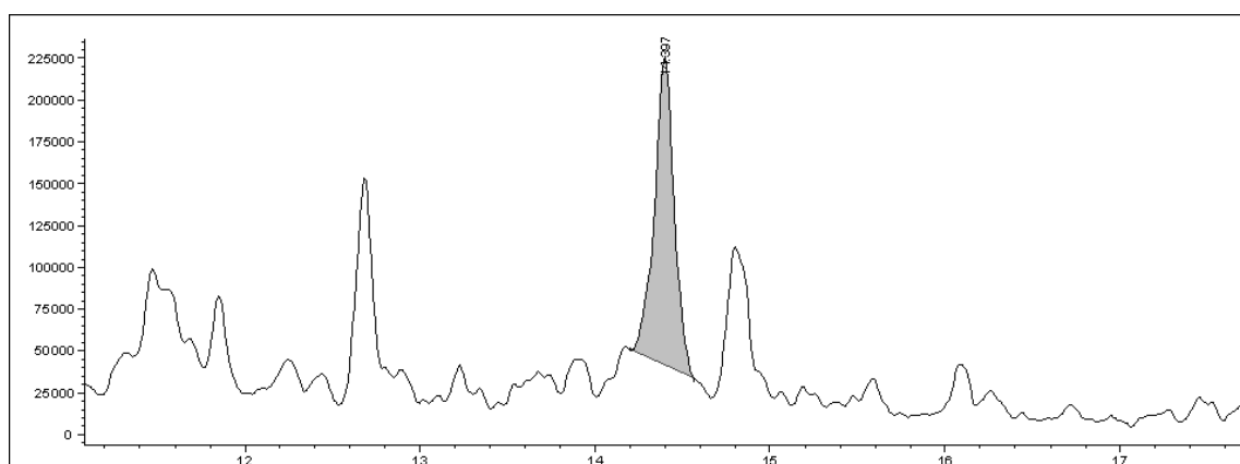
Figura 30 – Cromatogramma relativo all'estrazione dello ione 205 (Ibuprofen, 48 ng/L) del campione prelevato nel punto 4 in primavera.
