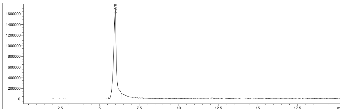
Figura 18 – Cromatogramma dello standard alla concentrazione equivalente a 500 ng/L in acqua per l'atenololo.
