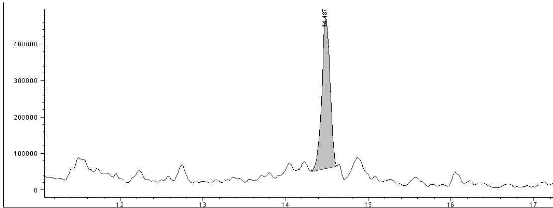
Figura 26 – Cromatogramma relativo all'estrazione dello ione 205 (Ibuprofen, 95 ng/L) del campione prelevato nel punto 3 in inverno.
