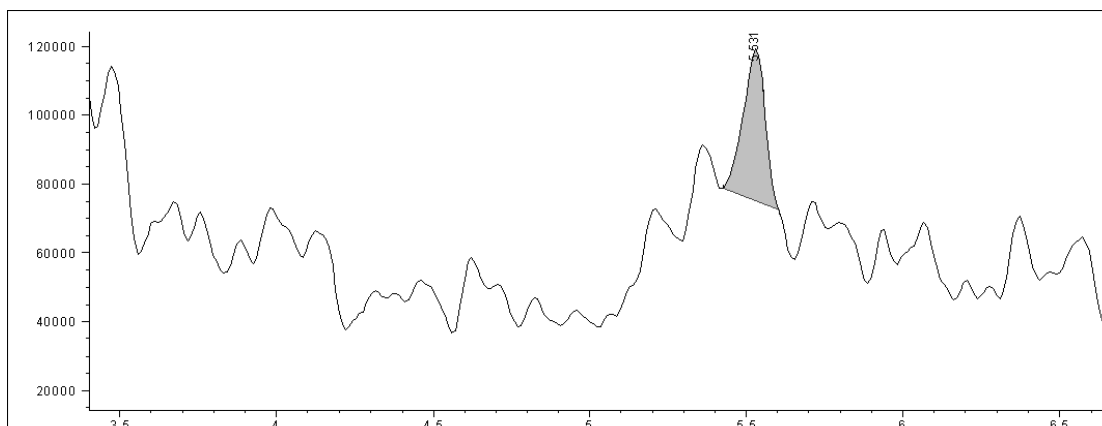
Figura 25 – Cromatogramma relativo all'estrazione degli ioni 296 e 298 (Idroclorotiazide, 18 ng/L) del campione prelevato nel punto 3 in inverno.
