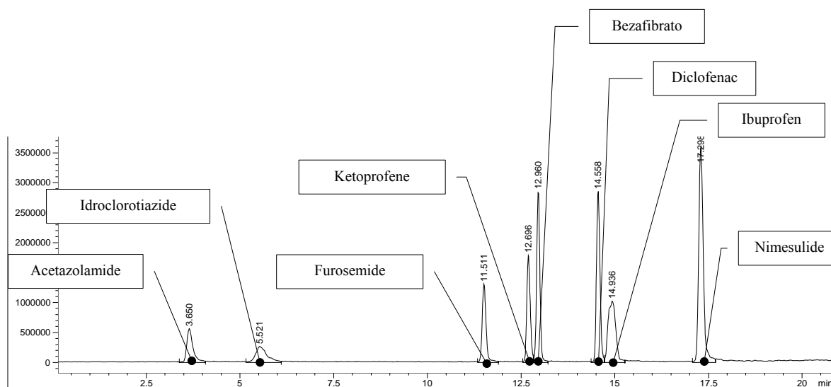
Figura 17 – Cromatogramma dello standard alla concentrazione equivalente a 500 ng/L in acqua per le sostanze del gruppo 1 ad esclusione dell'atenololo.
