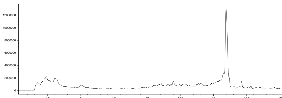
Figura 24 – Cromatogramma dello screening del campione prelevato nel punto 3 in inverno.
