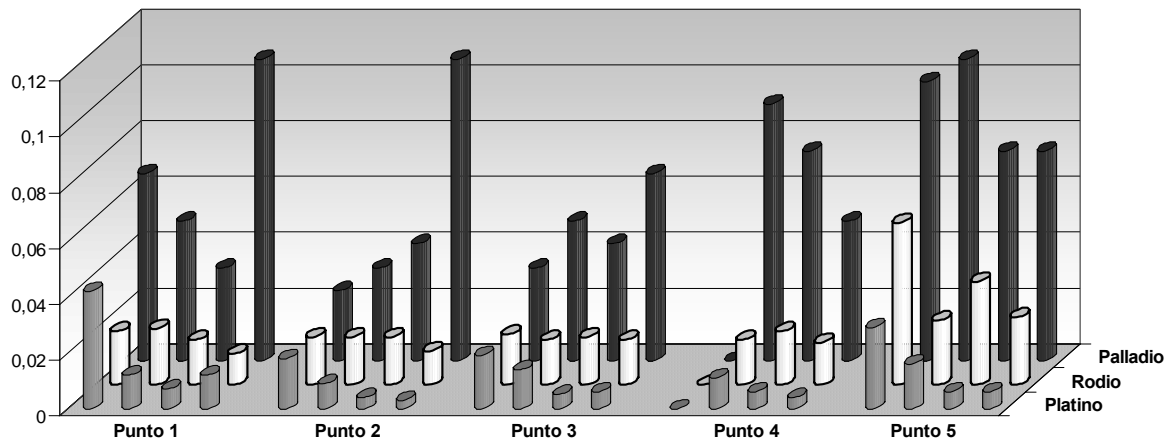
Grafico 9 – Andamento della concentrazione nelle 4 stagioni all'interno di uno stesso punto di prelievo dei metalli Pt, Pd e Rh detti PGEs ( Platinum Group Elements ).
