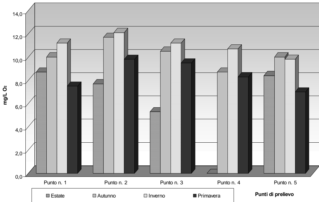
Grafico 3 - Andamento concentrazione O 2 libero per punti prelievo.
