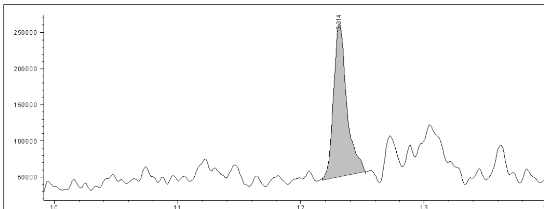
Figura 28 – Cromatogramma relativo all'estrazione degli ioni 294, 296 e 298 (Diclofenac, 33 ng/L) del campione prelevato nel punto 3 in inverno.
