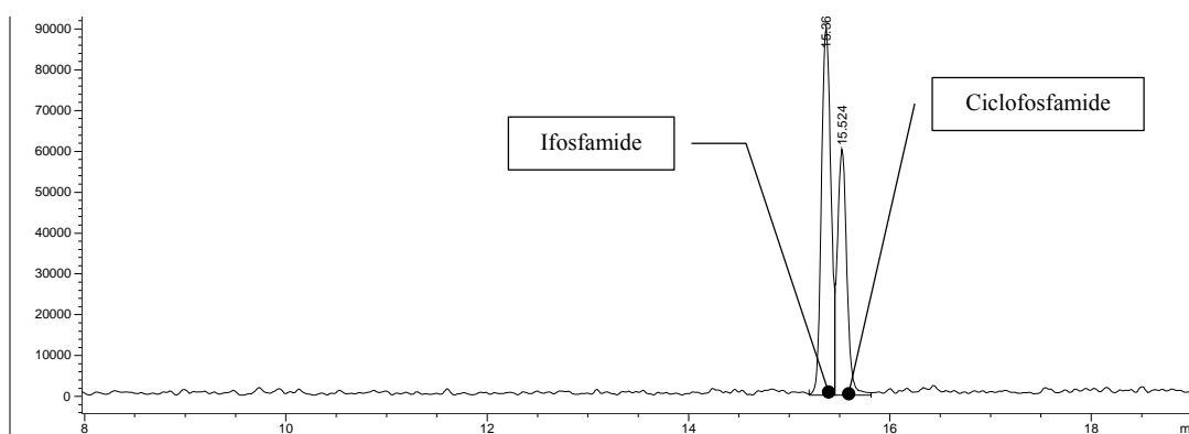
Figura 19 – Cromatogramma dello standard alla concentrazione equivalente a 500 ng/L in acqua per le sostanze del gruppo 2 ad esclusione del 5-fluorouracile.
