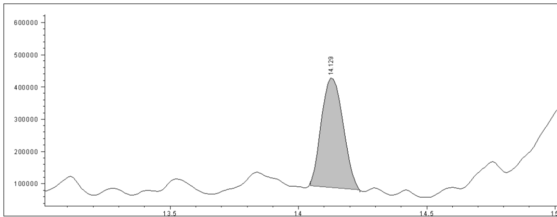
Figura 27 – Cromatogramma relativo all'estrazione dello ione 253 (Ketoprofene, 35 ng/L) del campione prelevato nel punto 3 in inverno.
