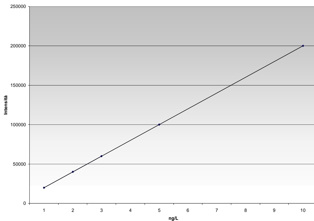
Figura 21 – Retta di taratura per il Platino.
