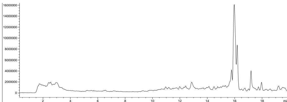
Figura 29 – Cromatogramma dello screening del campione prelevato nel punto 4 in primavera.
