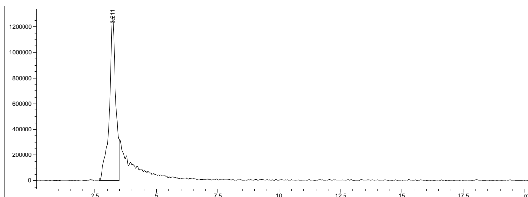
Figura 20 – Cromatogramma dello standard alla concentrazione equivalente a 500 ng/L in acqua per il 5-fluorouracile.
