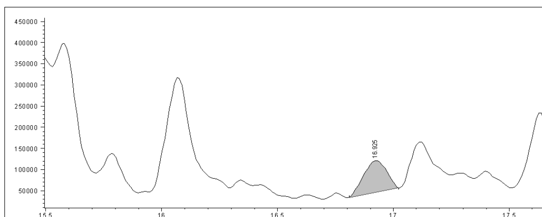
Figura 31 – Cromatogramma relativo all'estrazione dello ione 307 (Nimesulide, 5,2 ng/L) del campione prelevato nel punto 4 in primavera.
