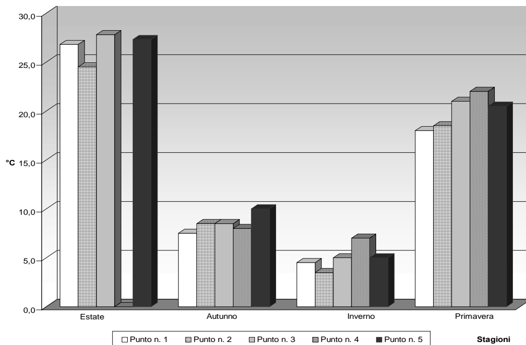
Grafico 5 - Andamento della temperatura.
